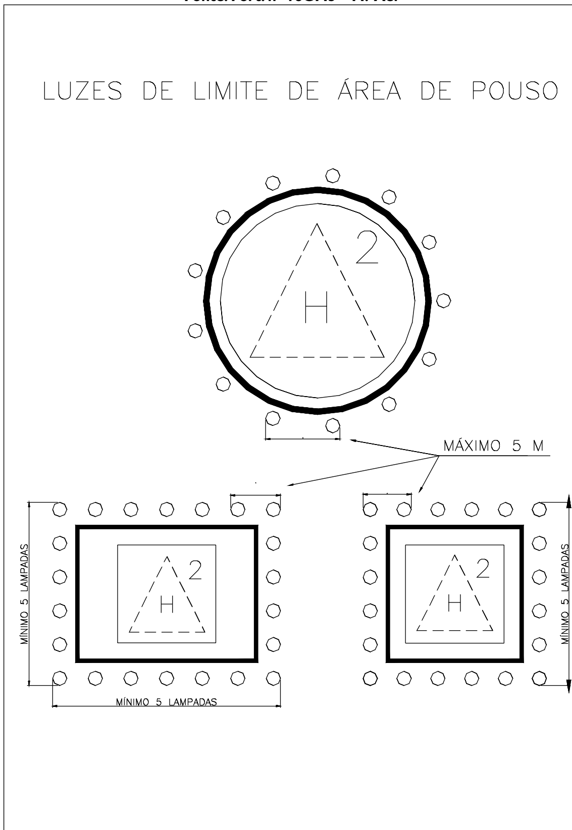
Figura 13: Luzes de limite para área de pouso
