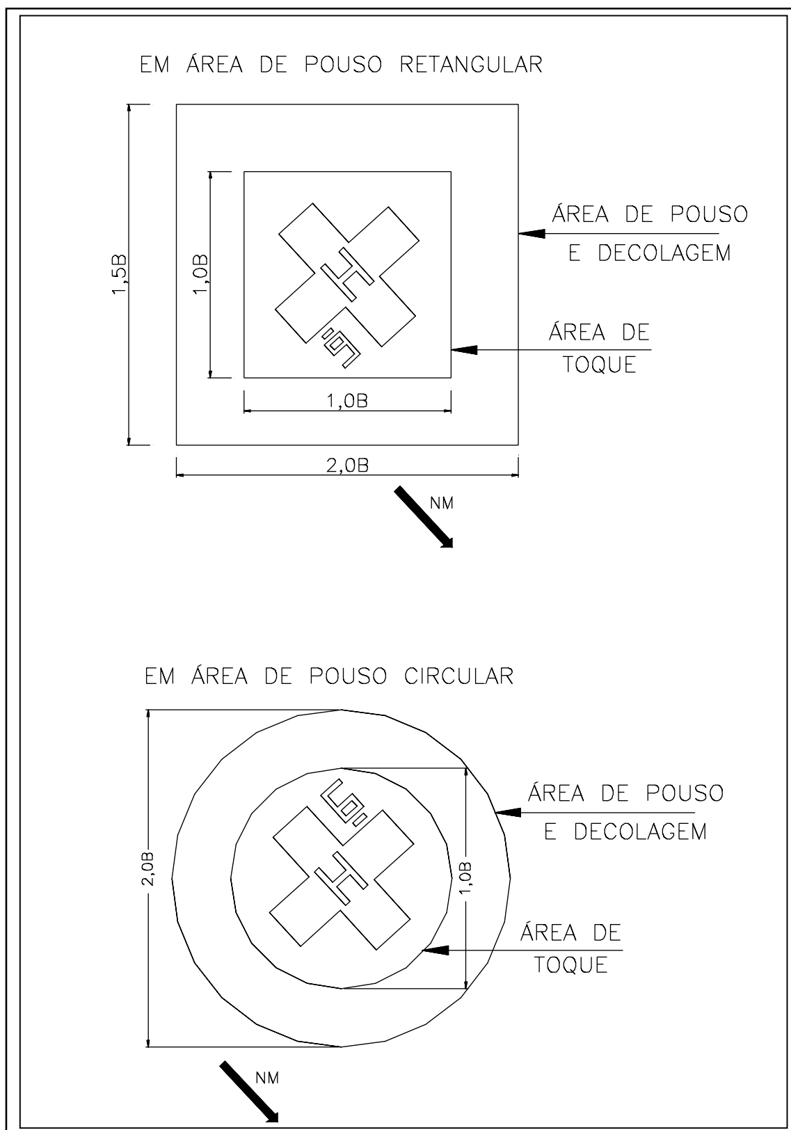
Figura I: Áreas de pouso e decolagem e áreas de toque
