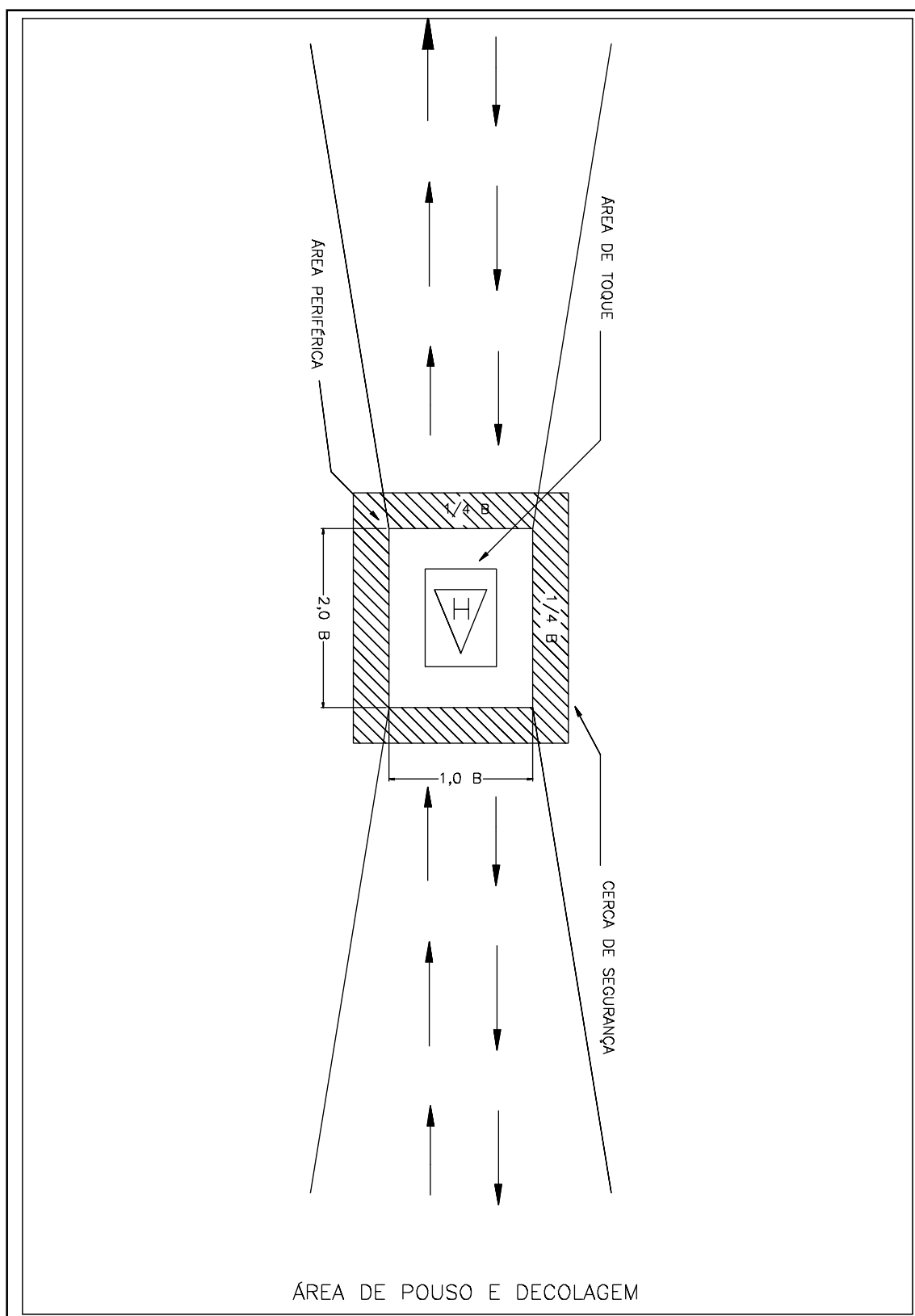
Anexo B: Figuras e modelos Figura 2: Área periférica e cerca de segurança Fonte: Port. nº 18GM5 – M. Aer
