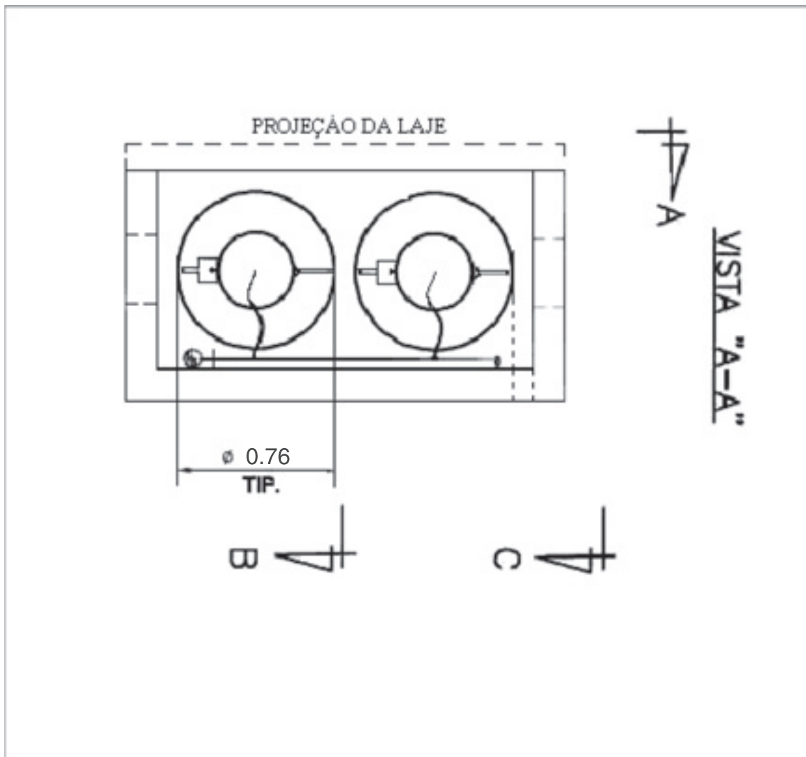
Planta baixa da central de GLP
