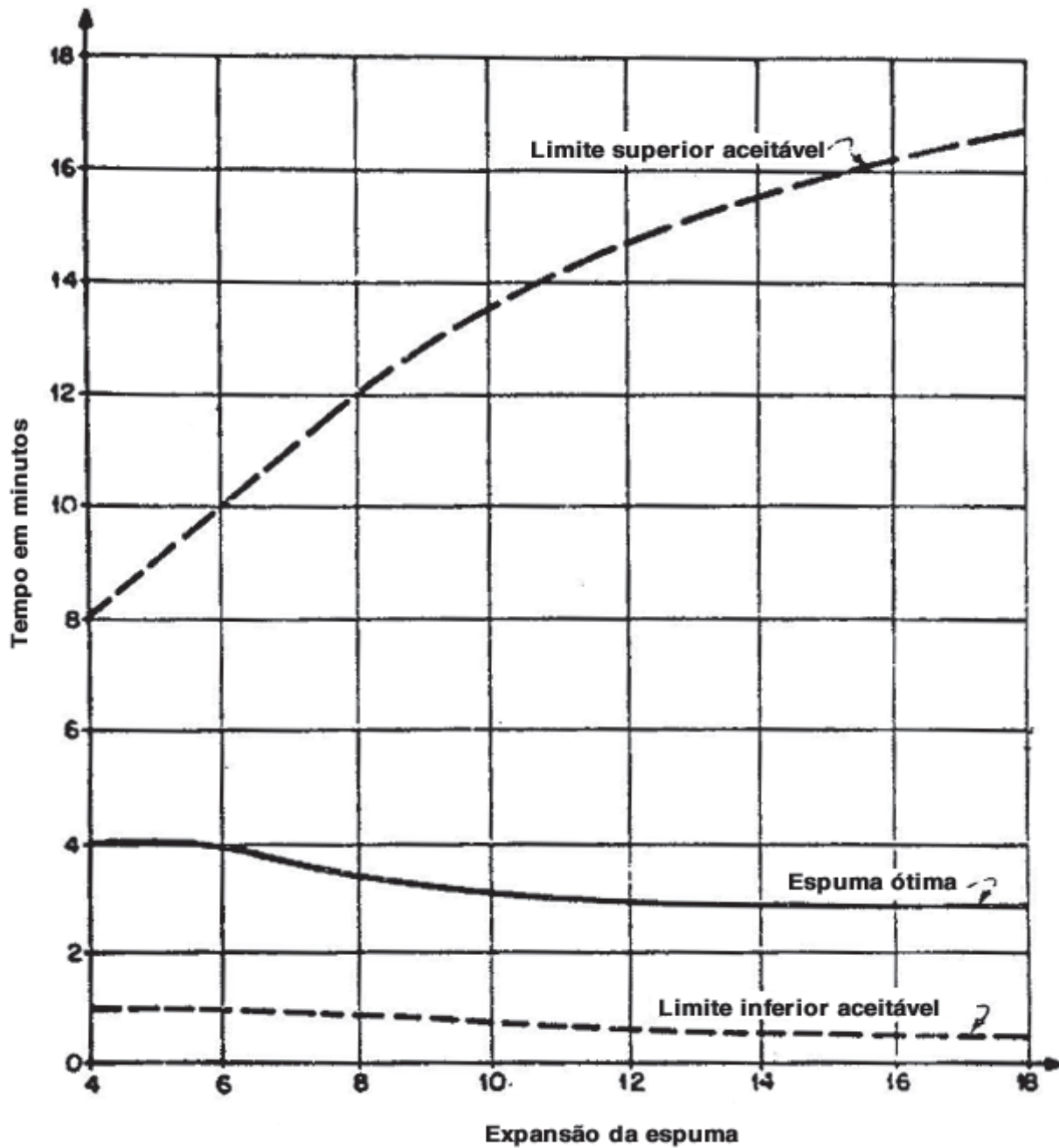
Figura I - Guia de qualidade da espuma para tanques de armazenamento
