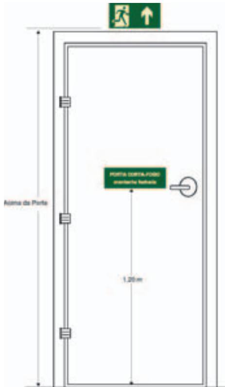
Figura 1 - Sinalização de porta corta-fogo (vista da escada)
