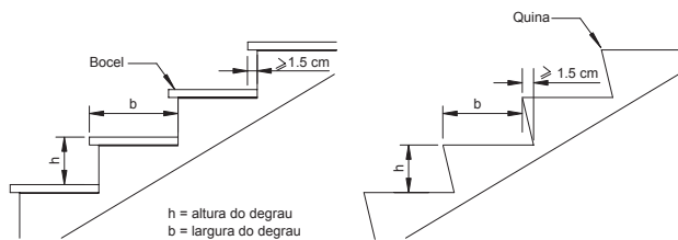
Figura 4 - Altura e largura dos degraus
