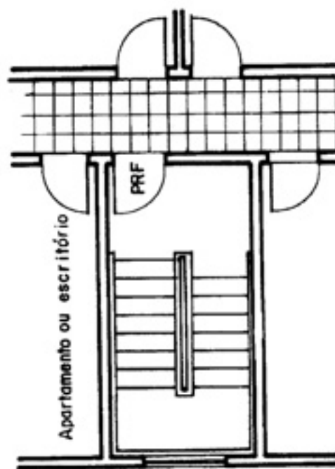
Figura 7 - Escada enclausurada protegida
