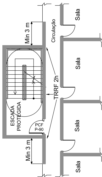
Figura 12 – Escada aberta externa
