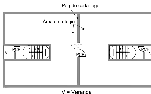
Figura 17 - Desenho esquemático da área de refúgio
