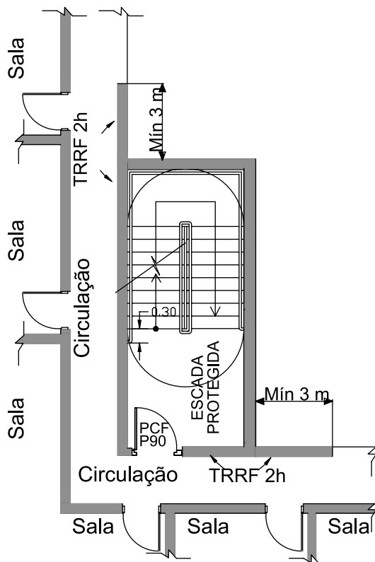
Figura 13 – Escada aberta externa
