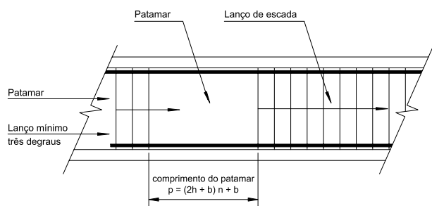
Figura 6 – Lanço mínimo e comprimento de patamar
