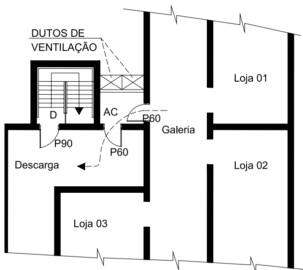
Figura 20 - Acesso de galeria comercial à descarga
