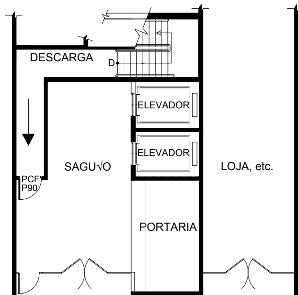
Figura 18 – Descarga através de hall térreo não enclausurado
