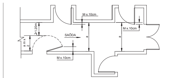
Figura 2 – Abertura das portas no sentido de saída
