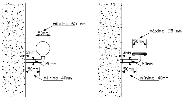
Figura 15 - Pormenores de corrimãos
