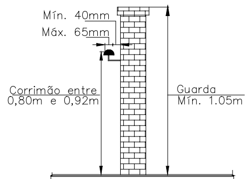
Figura 14 - Dimensões de guardas e corrimãos
