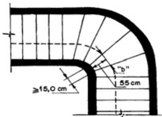
Figura 5 – Escada com lanços curvos e degraus balanceados
