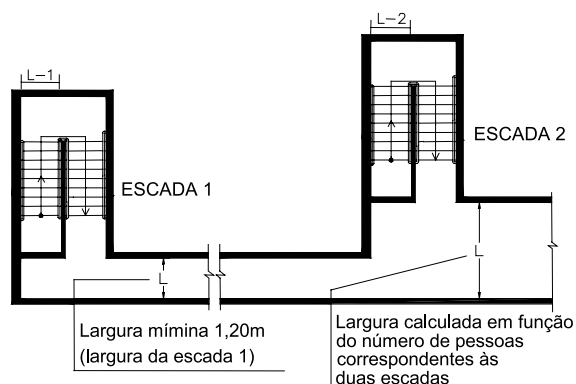
Figura 19 – Dimensionamento de corredores de descarga
