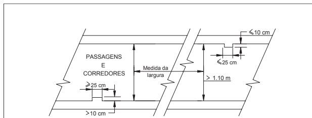
Figura 1 – Medida da largura em corredores e passagens
