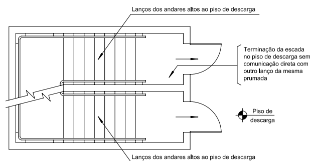
Figura 3 – Segmentação das escadas no piso da descarga
