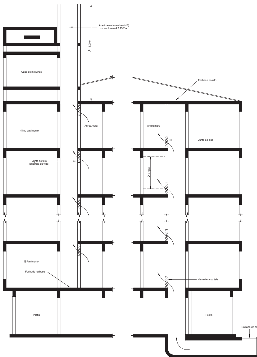
Figura 10 - Exemplo de dutos de ventilação
