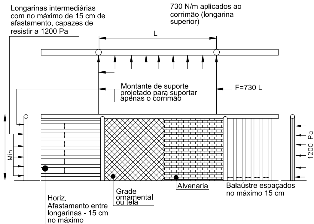
Figura 16 – Pormenores construtivos da instalação de guardas e as cargas a que elas devem resistir
